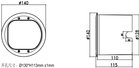
开孔尺寸: Ø130*H113mm ±1mm
